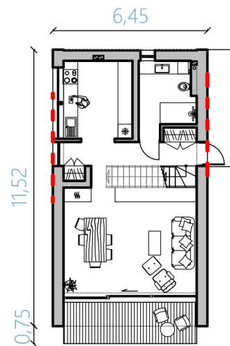
Pow. użytkowa parteru: 49,00 m 2
