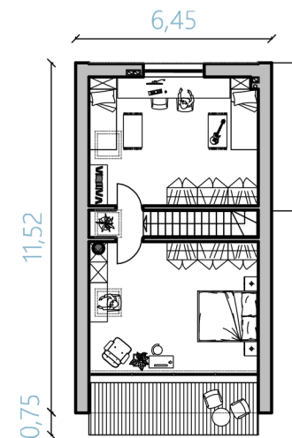
Pow. użytkowa poddasza (po podłodze): 47,30 m 2
