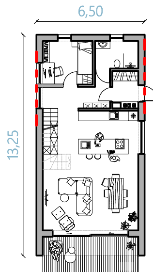
Pow. użytkowa parteru: 59,60 m 2
